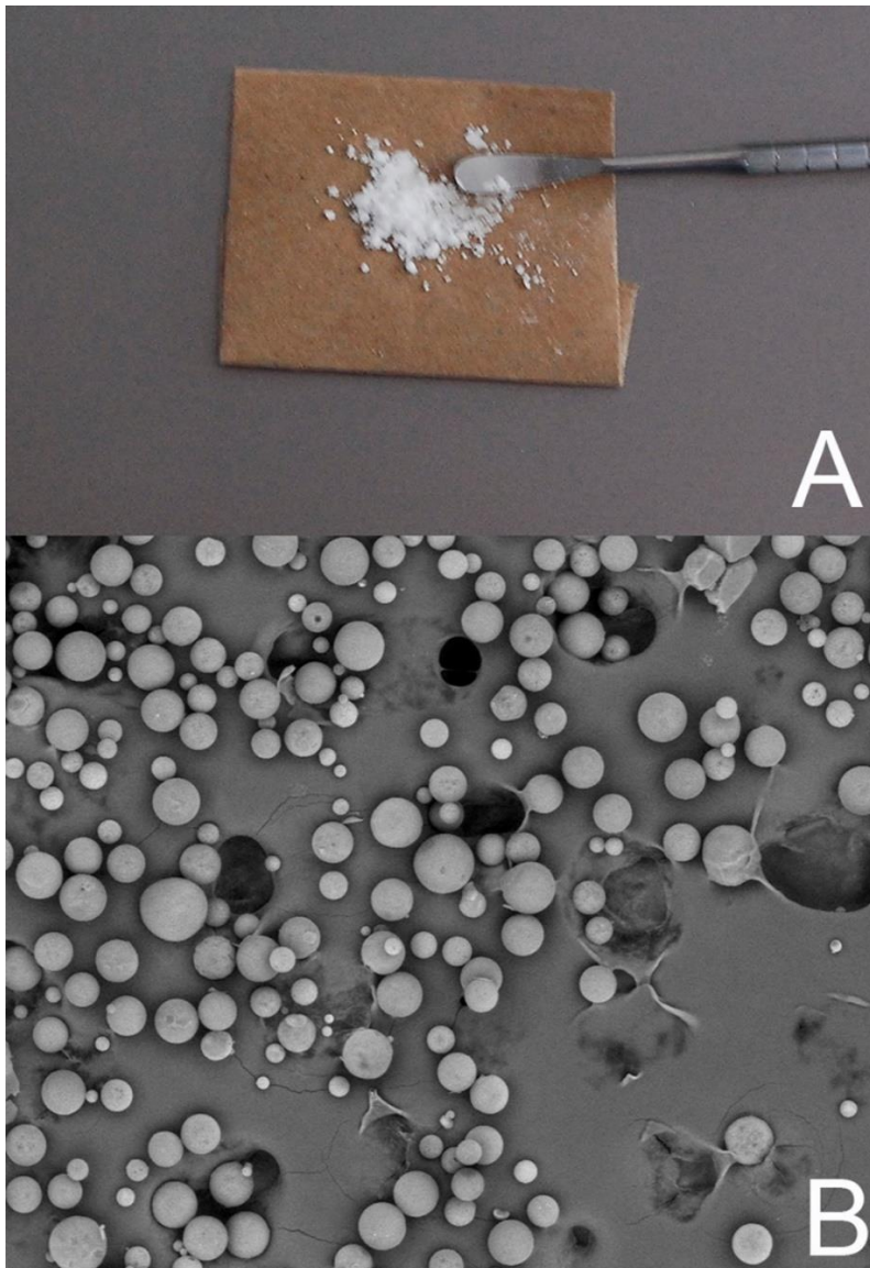
Figura 1. A) Vista macroscópica de las nanopartículas, se muestran como un polvo extrafino. B) Partículas de APLG con un rango de tamaño de 500-1000 nm.
